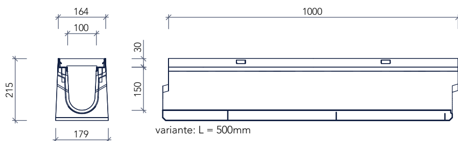
vooraanzicht & langsdoorsnede
