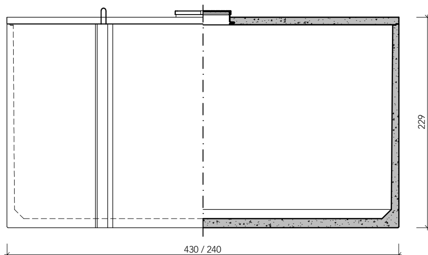
zijaanzicht / doorsnede
