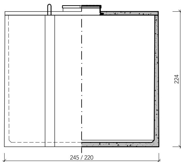
zijaanzicht / doorsnede
