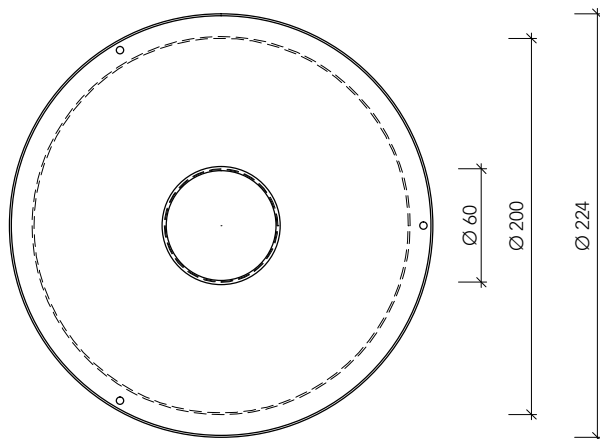
bovenaanzicht
