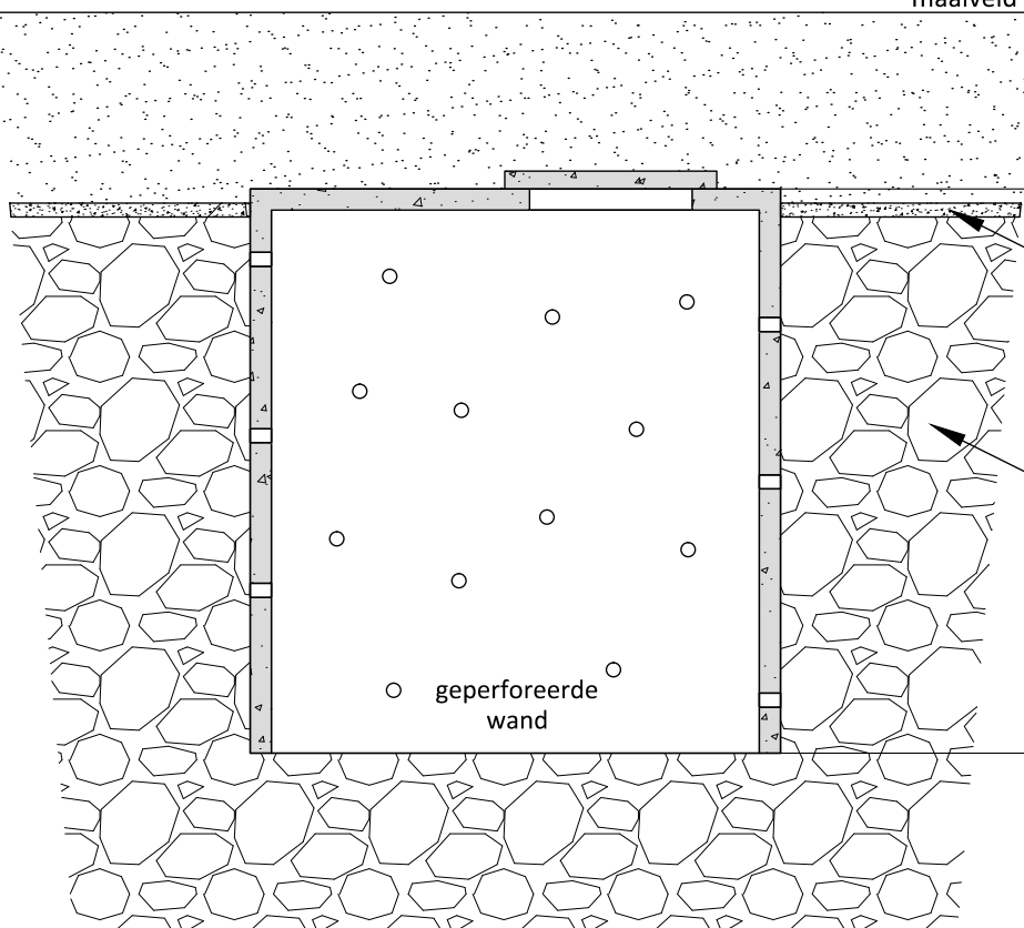
doorsnede
