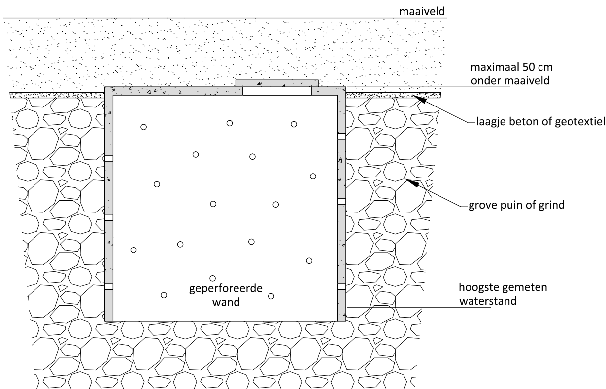
doorsnede
