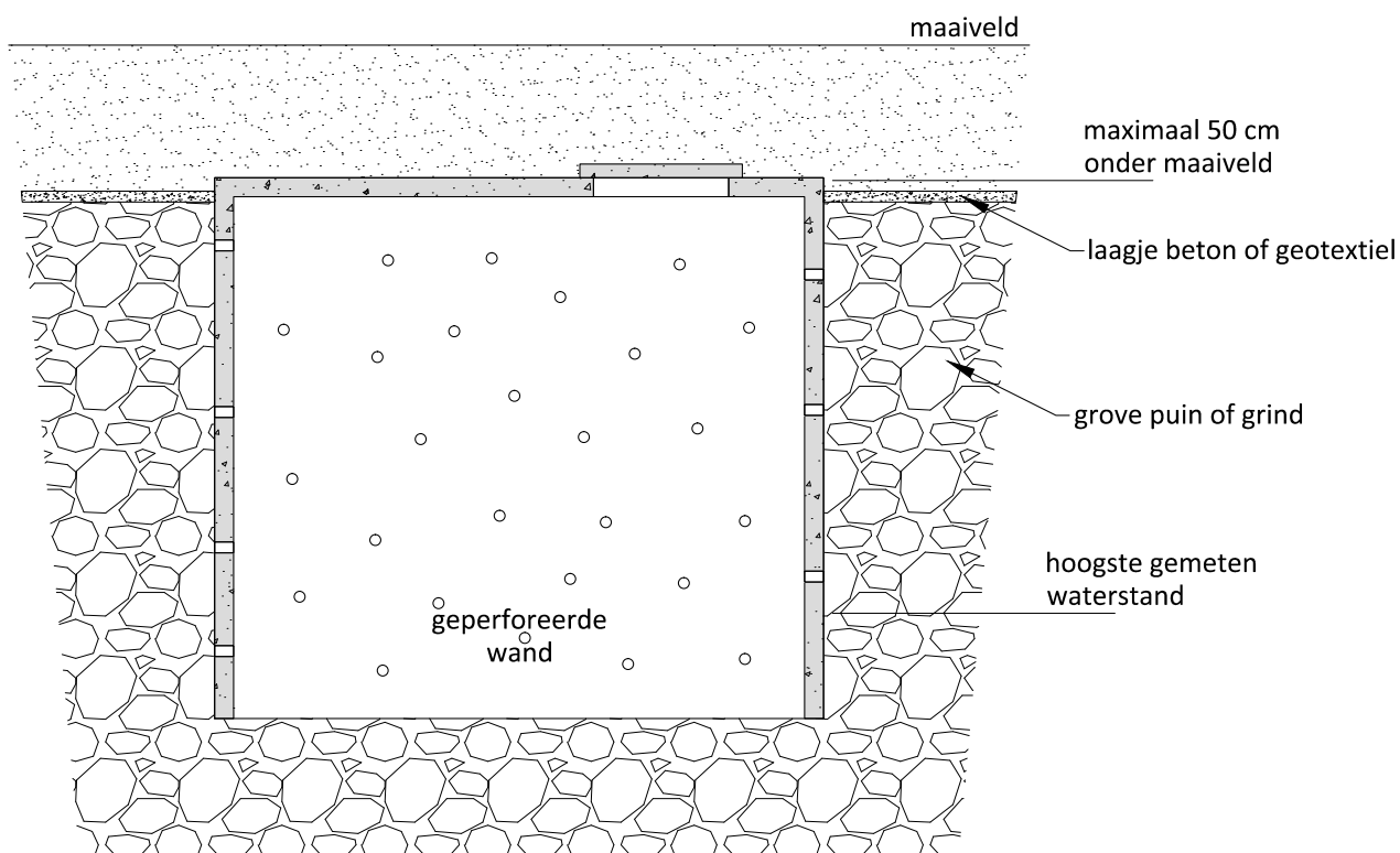
doorsnede
