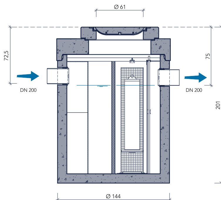
doorsnede
