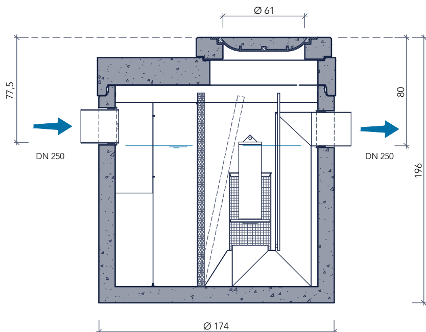
doorsnede
