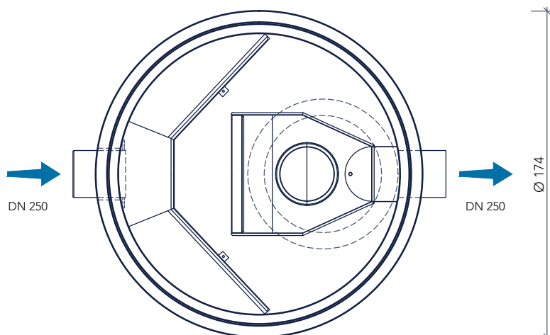
bovenaanzicht
