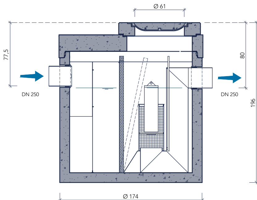
doorsnede
