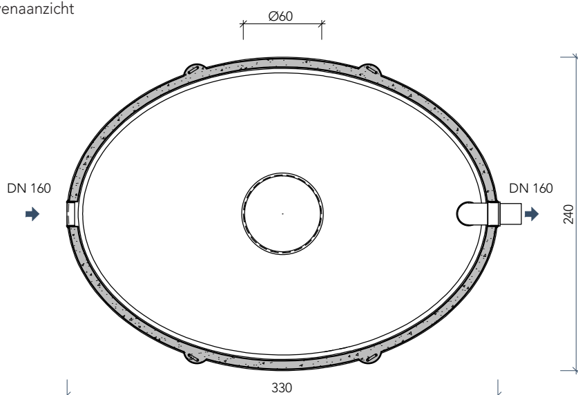
bovenaanzicht
