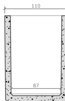
dwarse doorsnede
