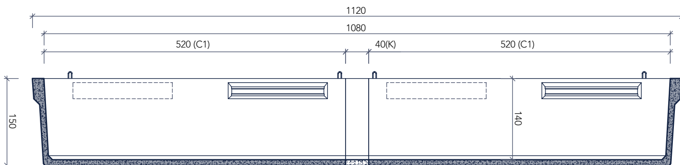
langse doorsnede
