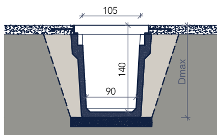
dwarse doorsnede
