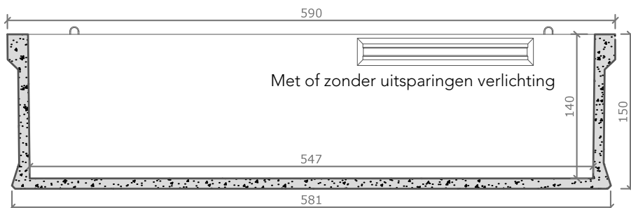
langse doorsnede
