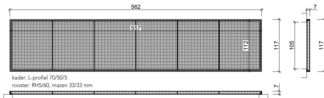
gegalvaniseerd kader & rooster leverbaar in verkeersklasse A, B, C & D
