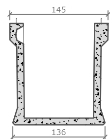
dwarse doorsnede
