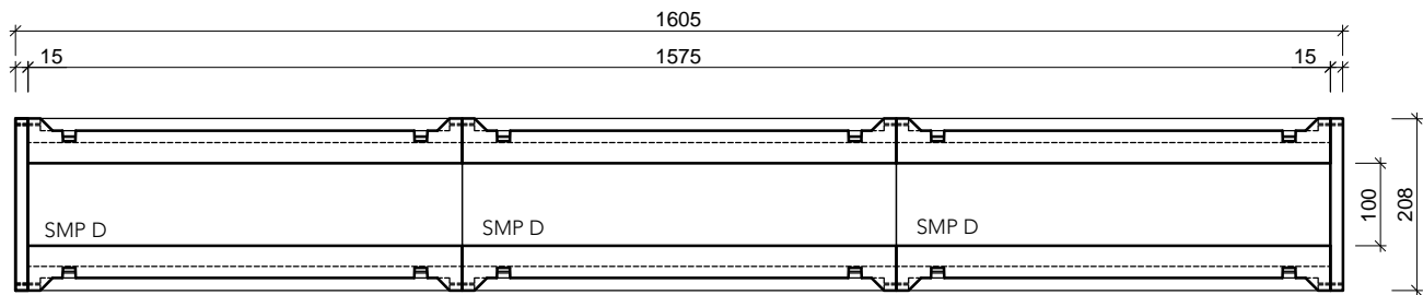
bovenaanzicht
