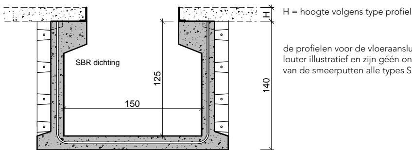
dwarsdoorsnede
