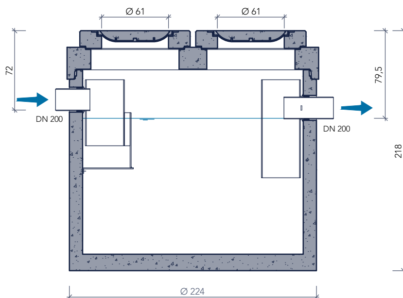
doorsnede
