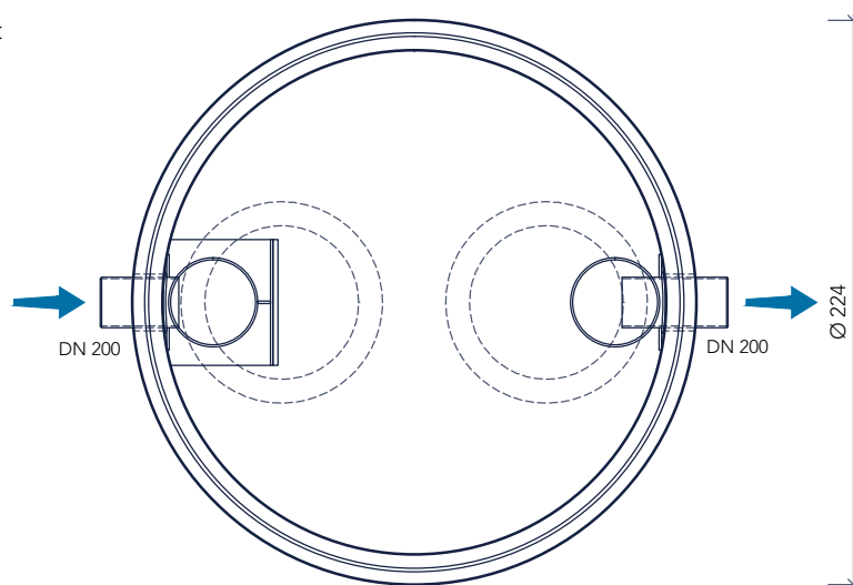
bovenaanzicht
