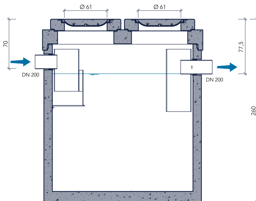
doorsnede
