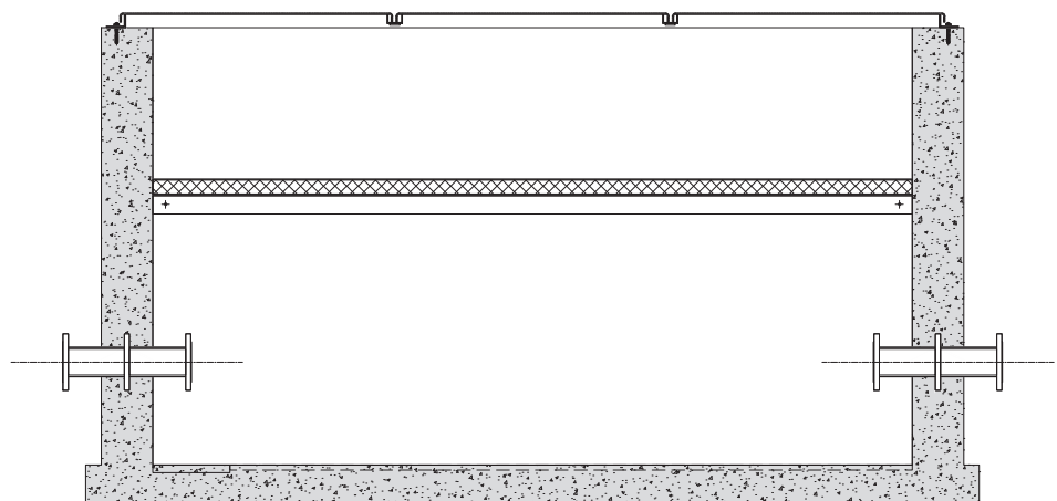
Doorsnede
