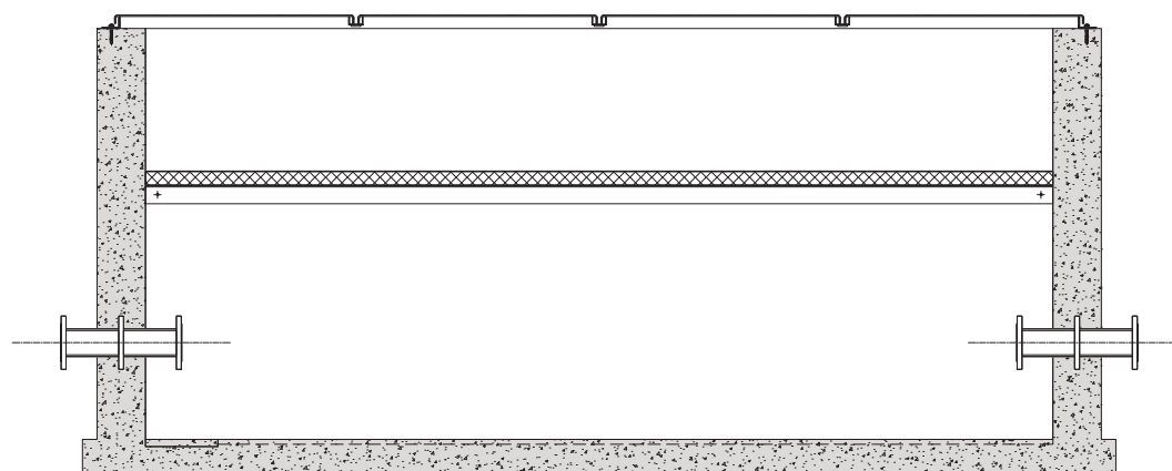
Doorsnede
