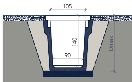
dwarse doorsnede
