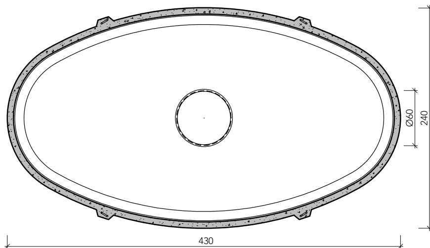
bovenaanzicht
