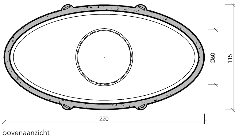
bovenaanzicht
