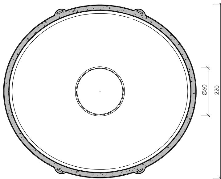
bovenaanzicht
