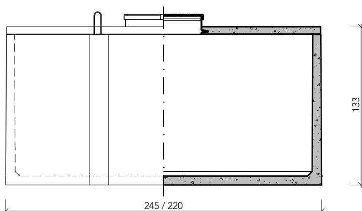
zijaanzicht / doorsnede
