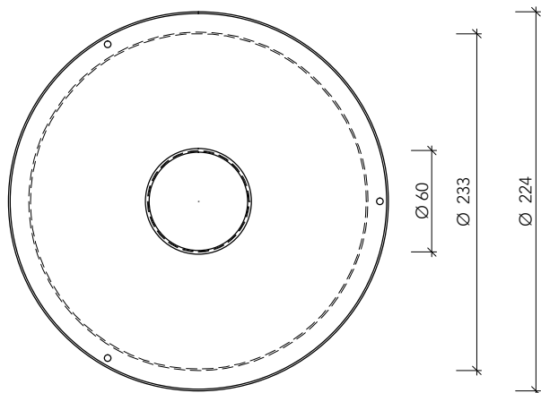
bovenaanzicht
