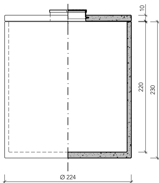
zijaanzicht / doorsnede
