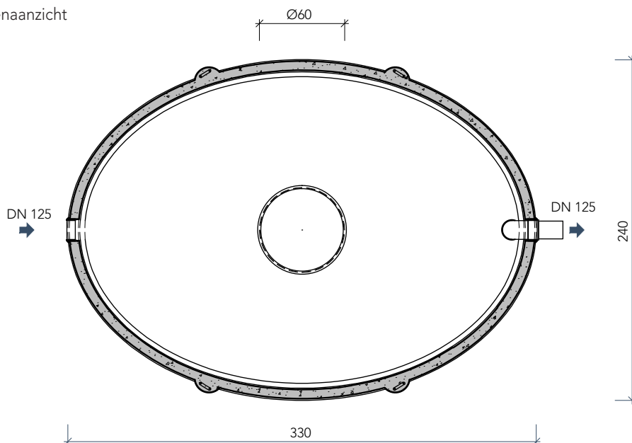
bovenaanzicht
