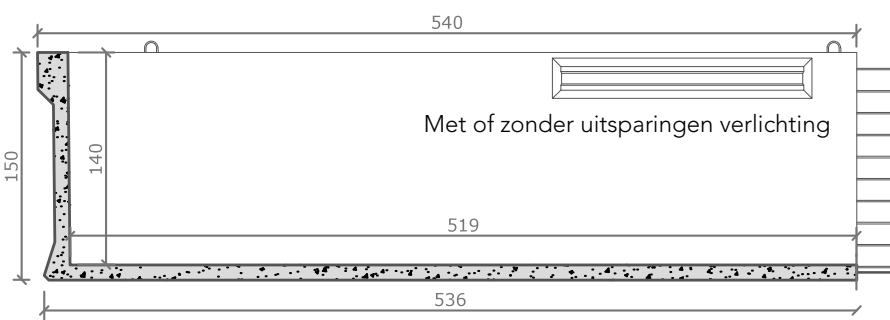
langse doorsnede
