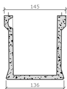
dwarse doorsnede
