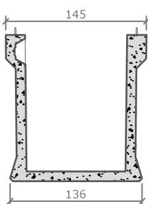
dwarse doorsnede
