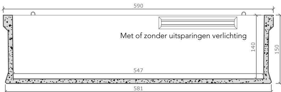
langse doorsnede
