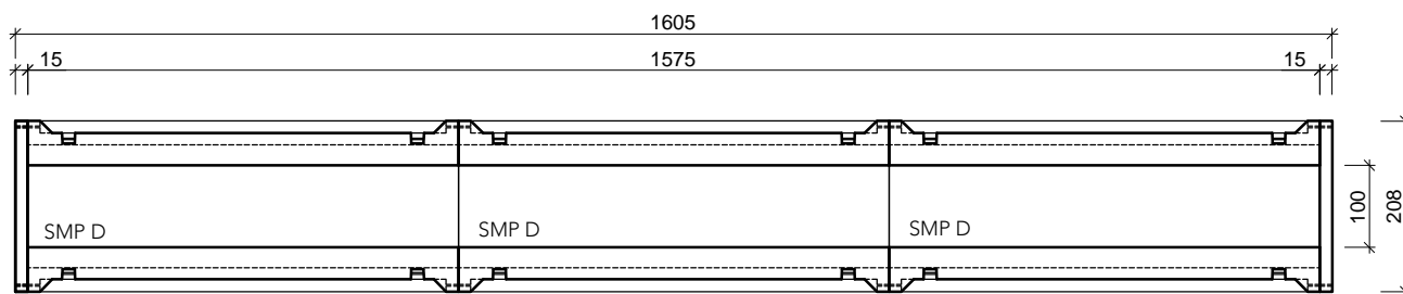
bovenaanzicht
