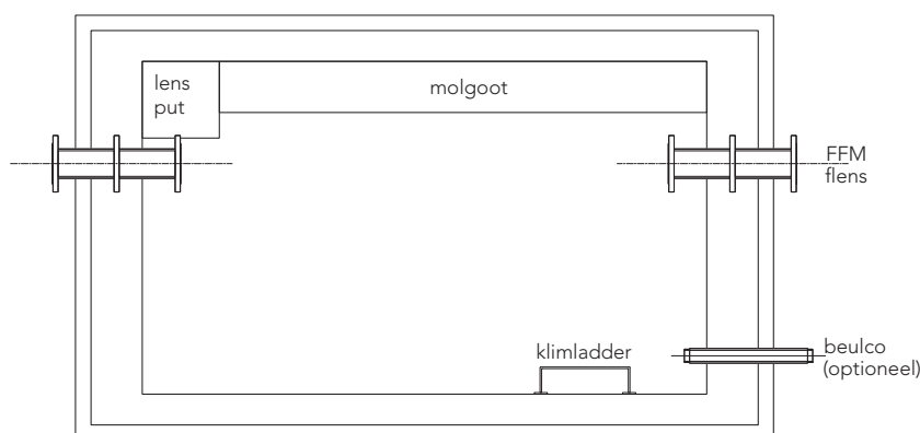
Bovenaanzicht put
