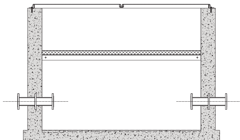
Doorsnede
