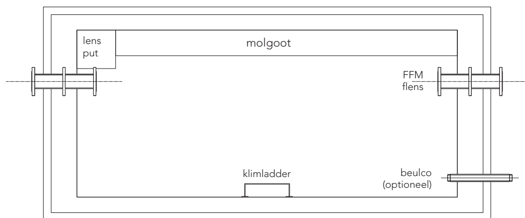
Bovenaanzicht put
