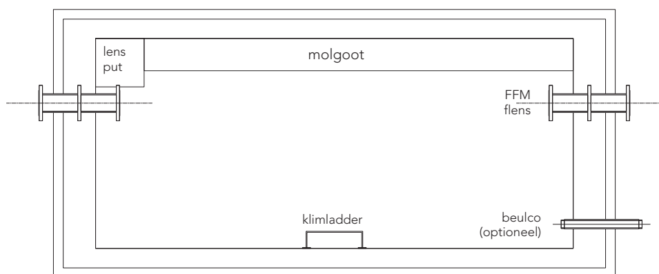
Bovenaanzicht put
