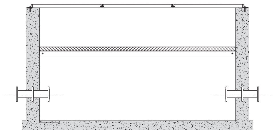
Doorsnede
