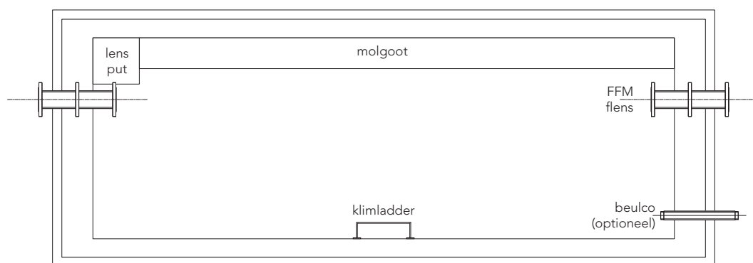
Bovenaanzicht put
