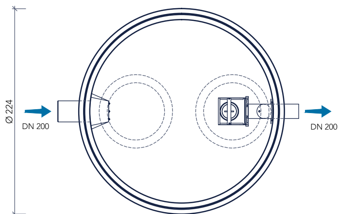
bovenaanzicht
