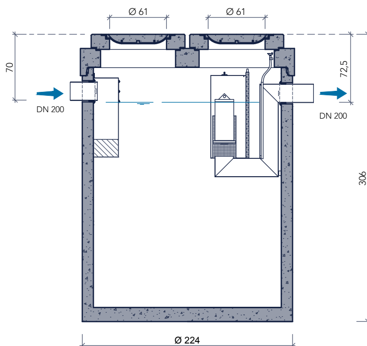
doorsnede
