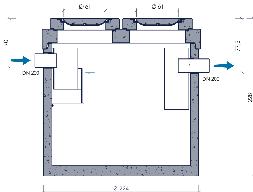
doorsnede
