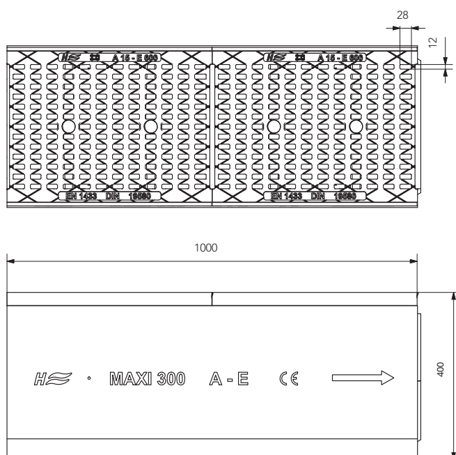
boven- en zijaanzicht 1000 mm
