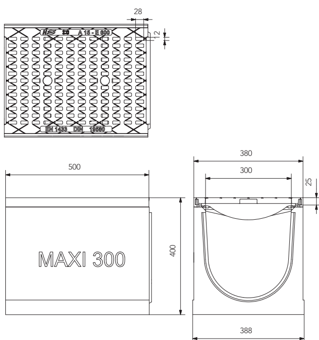
boven- en zijaanzicht 500 mm
