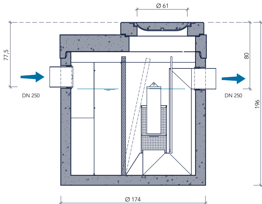
doorsnede
