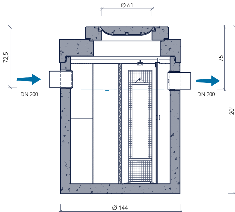
doorsnede
