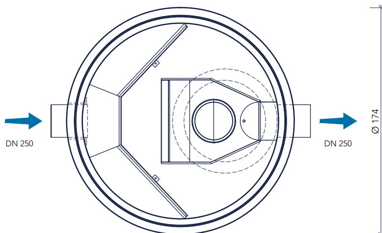
bovenaanzicht
