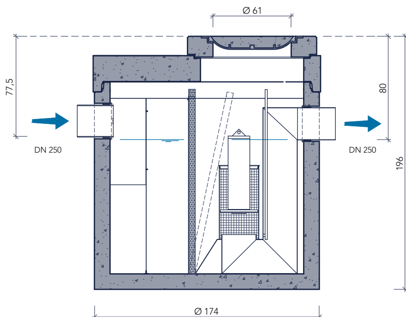
doorsnede
