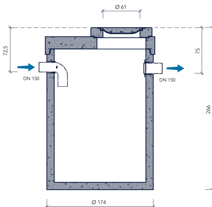
doorsnede
