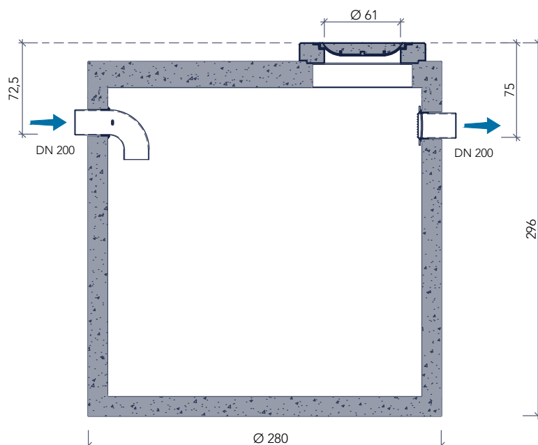
doorsnede
