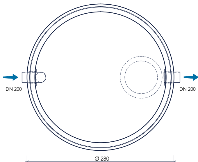
bovenaanzicht
