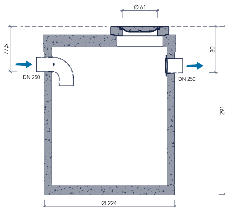
doorsnede
