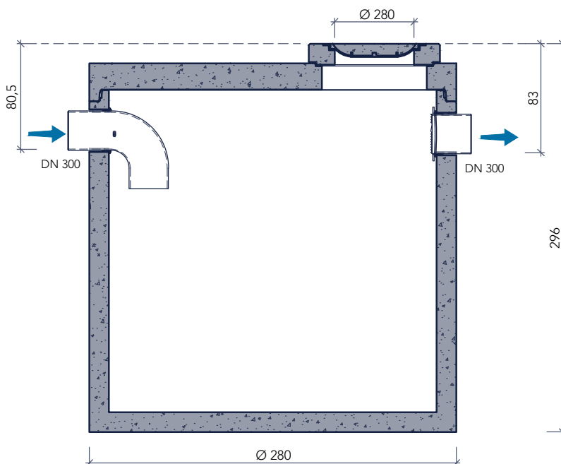
doorsnede
