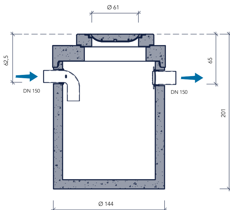
doorsnede
