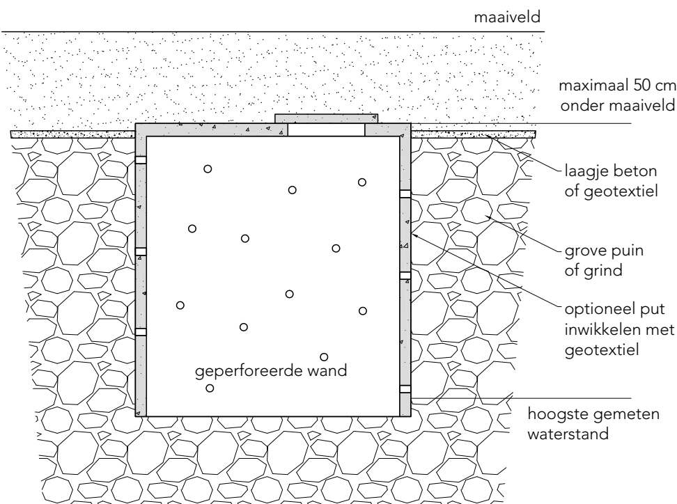
doorsnede
