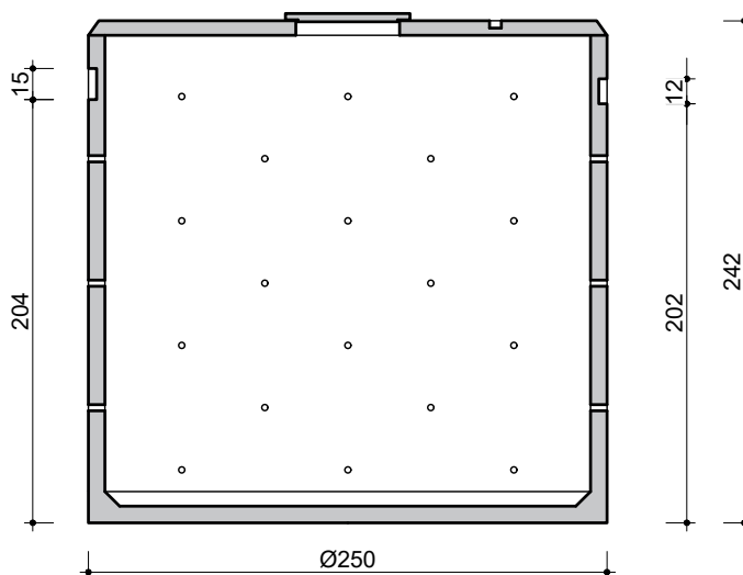
DOORSNEDE
