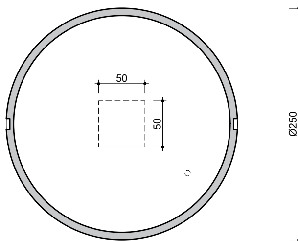
BOVENAANZICHT
