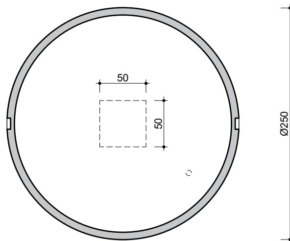
BOVENAANZICHT
