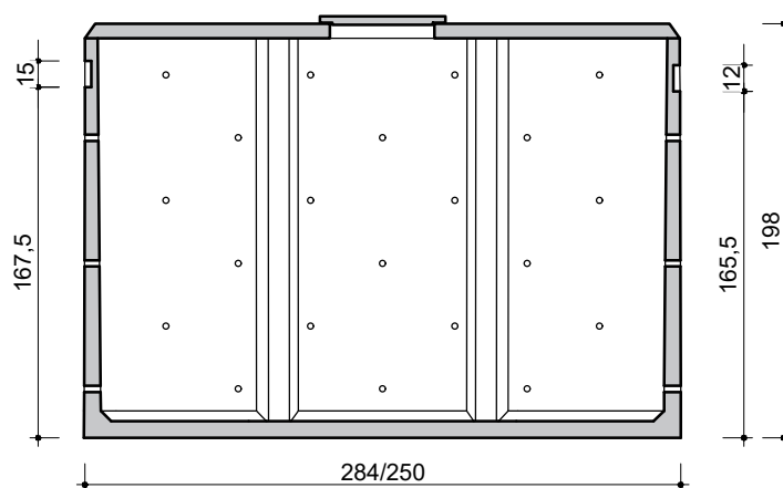
DOORSNEDE
