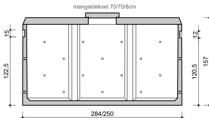
DOORSNEDE
