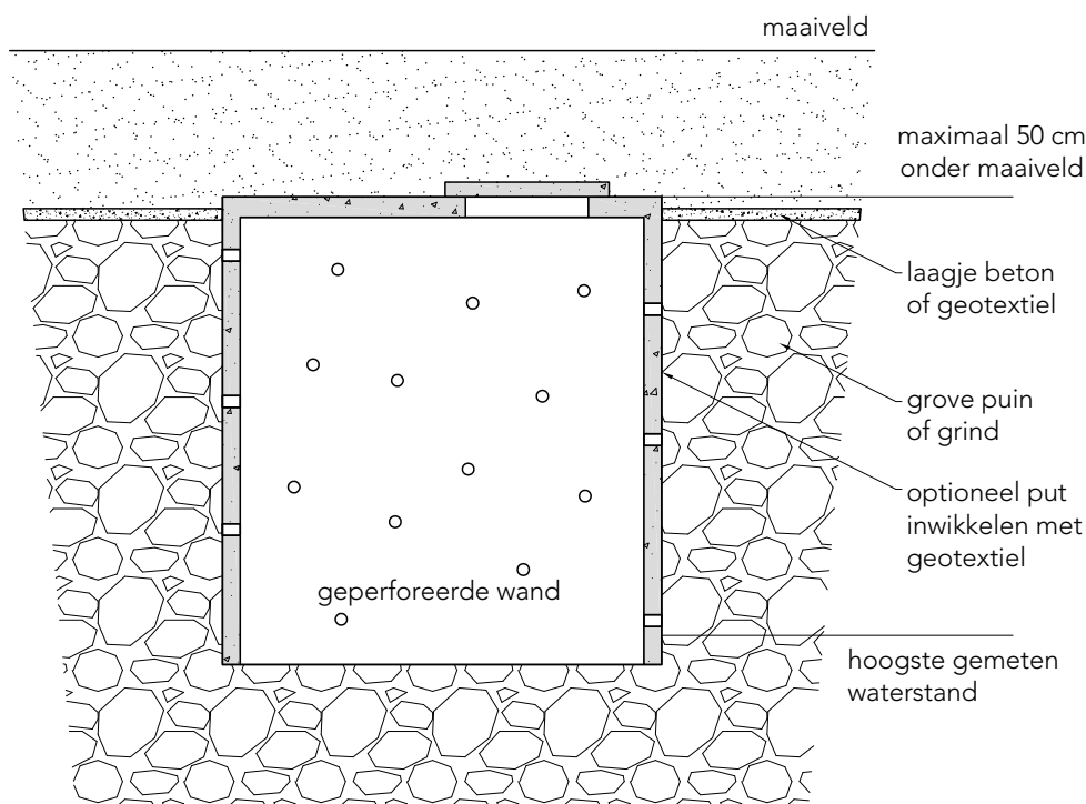
doorsnede
